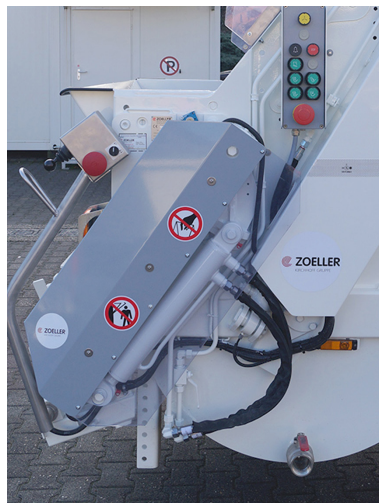
Schutzabdeckungen
